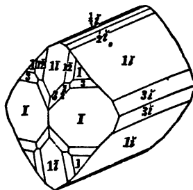
Danaite.
